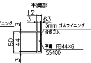
ゴムライニング部詳細図
